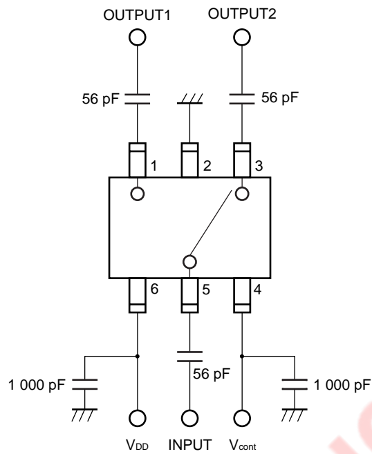
評価回路図 ( V_{DD} = 2.8\text{ V} , V_{cont} = 2.8\text{ V}/0\text{ V} , DC カット・コンデンサ = 56\text{ pF} )
