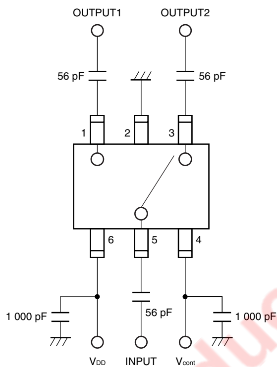
評価回路図 (V DD = 2.8 V, V cont = 2.8 V/0 V, DC カット・コンデンサ = 56 pF)
