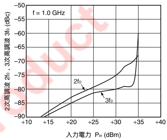
2次高調波, 3次高調波 vs. 入力電力
