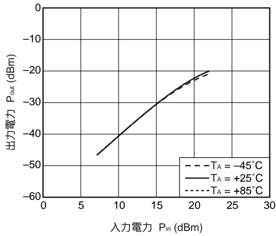
入出力特性の温度依存性
