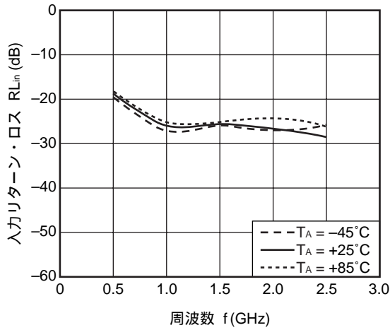
入力リターン・ロス vs. 周波数
