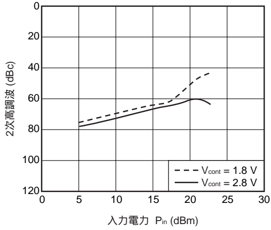
2次高調波の入力依存性
