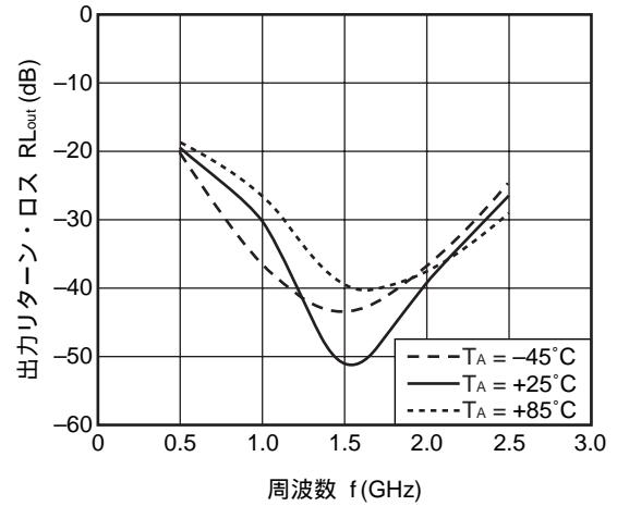
出力リターン・ロス vs. 周波数
