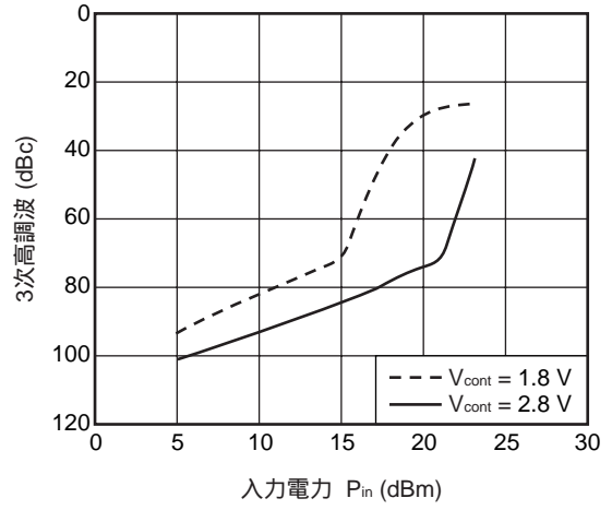
3次高調波の入力依存性
