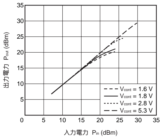
入出力特性の電圧依存性
