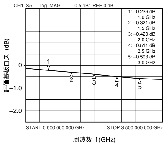
評価基板ロス vs. 周波数
