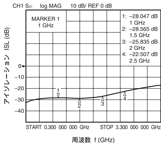
IN-OUT1 アイソレーション vs. 周波数
