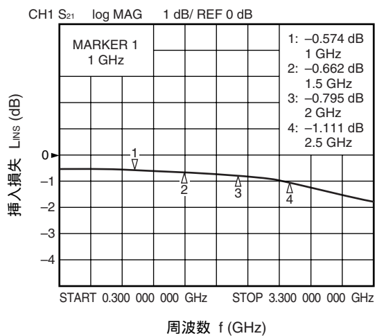
IN-OUT1 挿入損失 vs. 周波数
