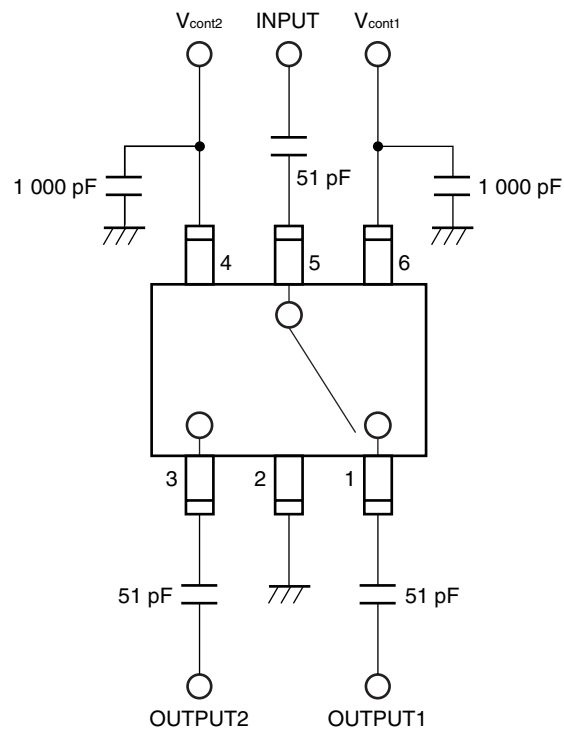
評価回路図 ( V_{cont} = 3.0\text{ V}/0\text{ V} , DC カット・コンデンサ = 51 pF)
