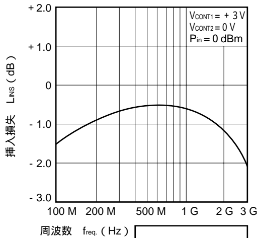
IN-OUT2 挿入損失 vs. 周波数
