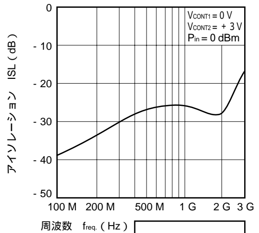
IN-OUT2 アイソレーション vs. 周波数
