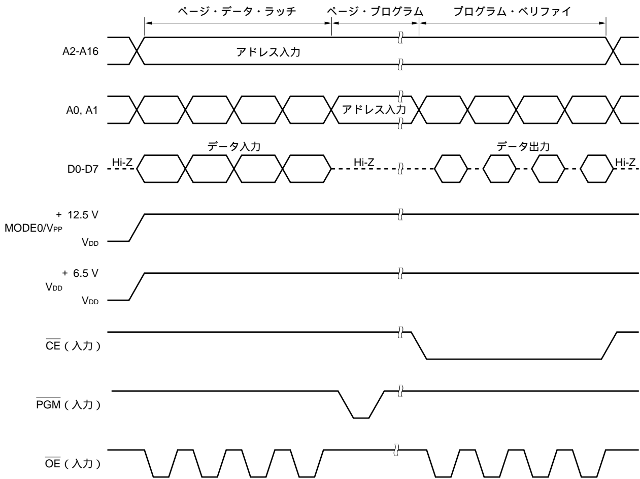
図4 - 2 PROMの書き込み/ペリファイ・タイミング(ページ・プログラム・モード)
