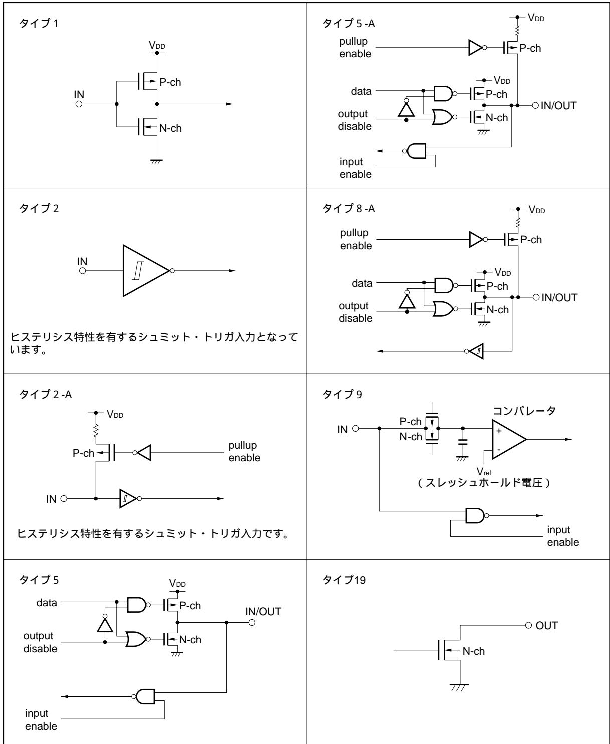
図1-1 端子の入出力回路
