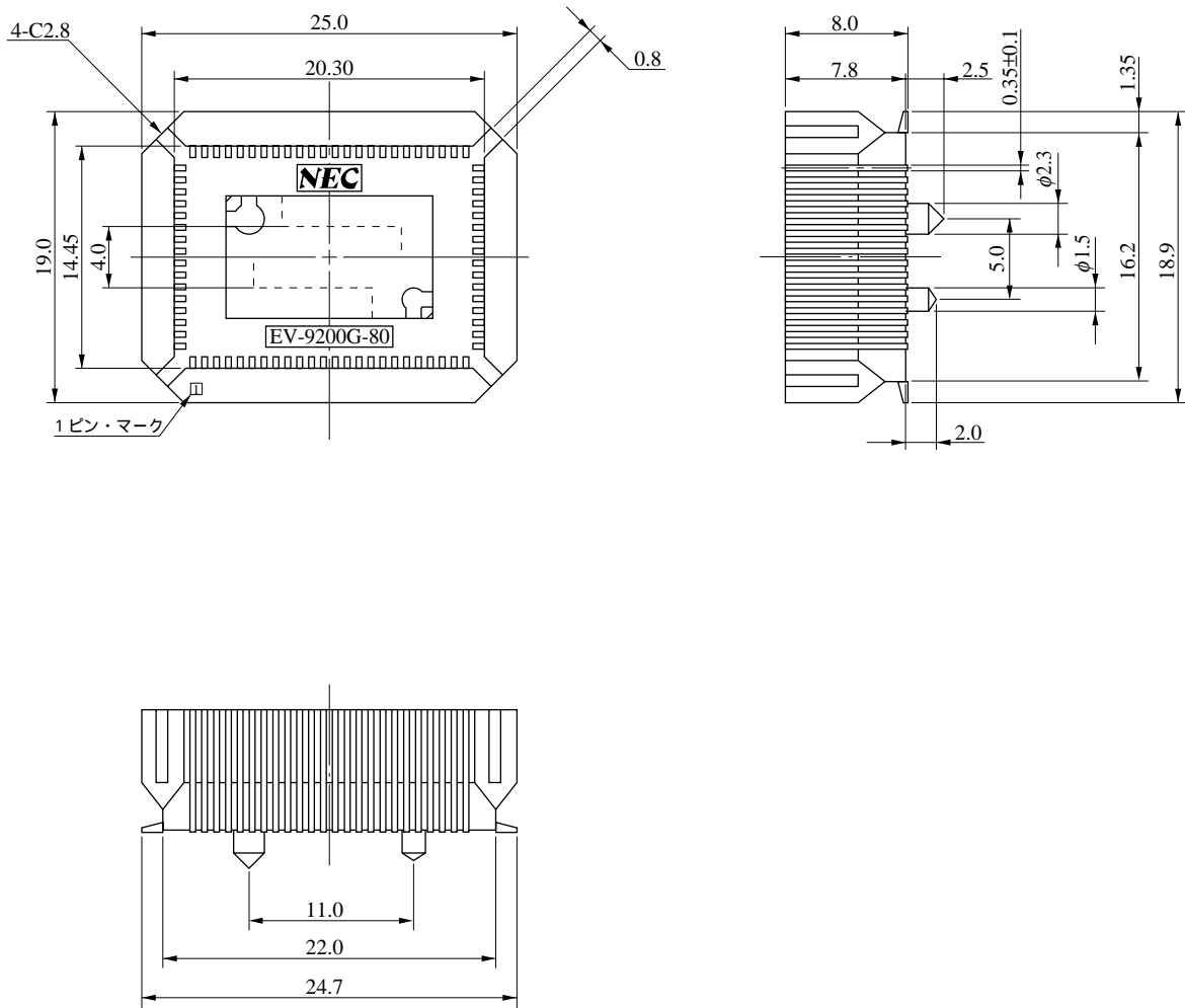
図B - 1 変換ソケット (EV-9200G-80) 外形図 (参考) (単位: mm)
