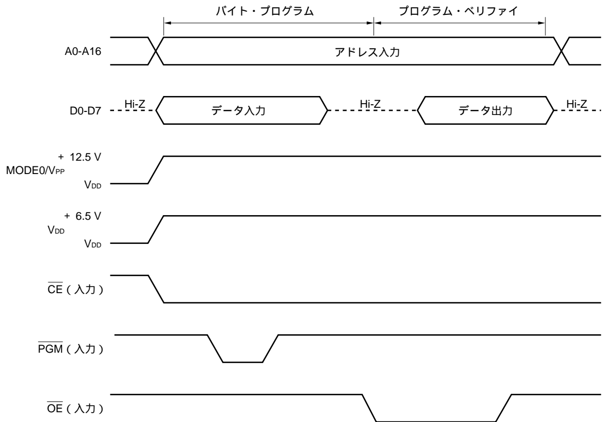
図4 - 4 PROMの書き込み/ベリファイ・タイミング (バイト・プログラム・モード)
