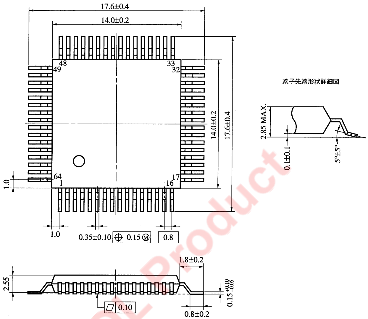
64ピン・プラスチック QFP (□14) 外形図 (単位: mm)
