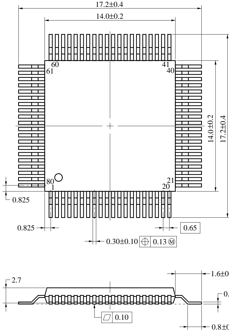
80ピン・プラスチック QFP (14×14) 外形図 (単位: mm)
