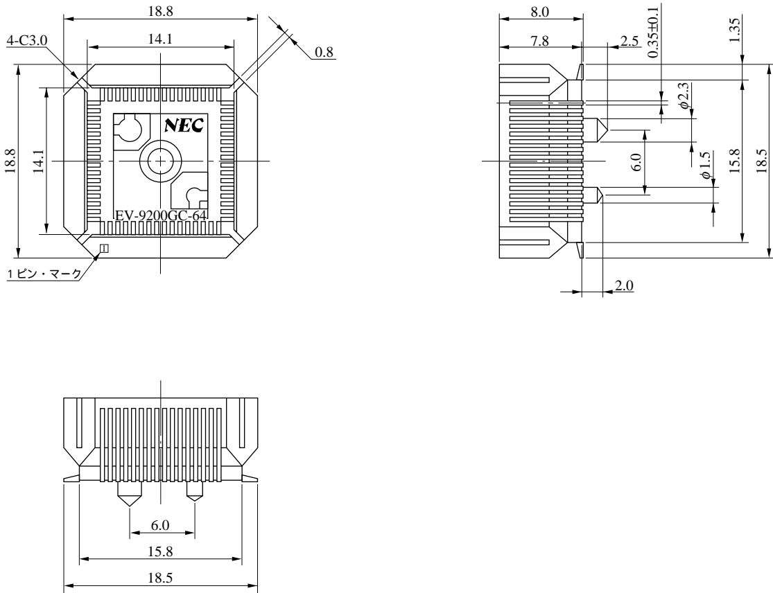
図 A - 1 EV-9200GC-64 外形図 (参考) (単位 : mm)
