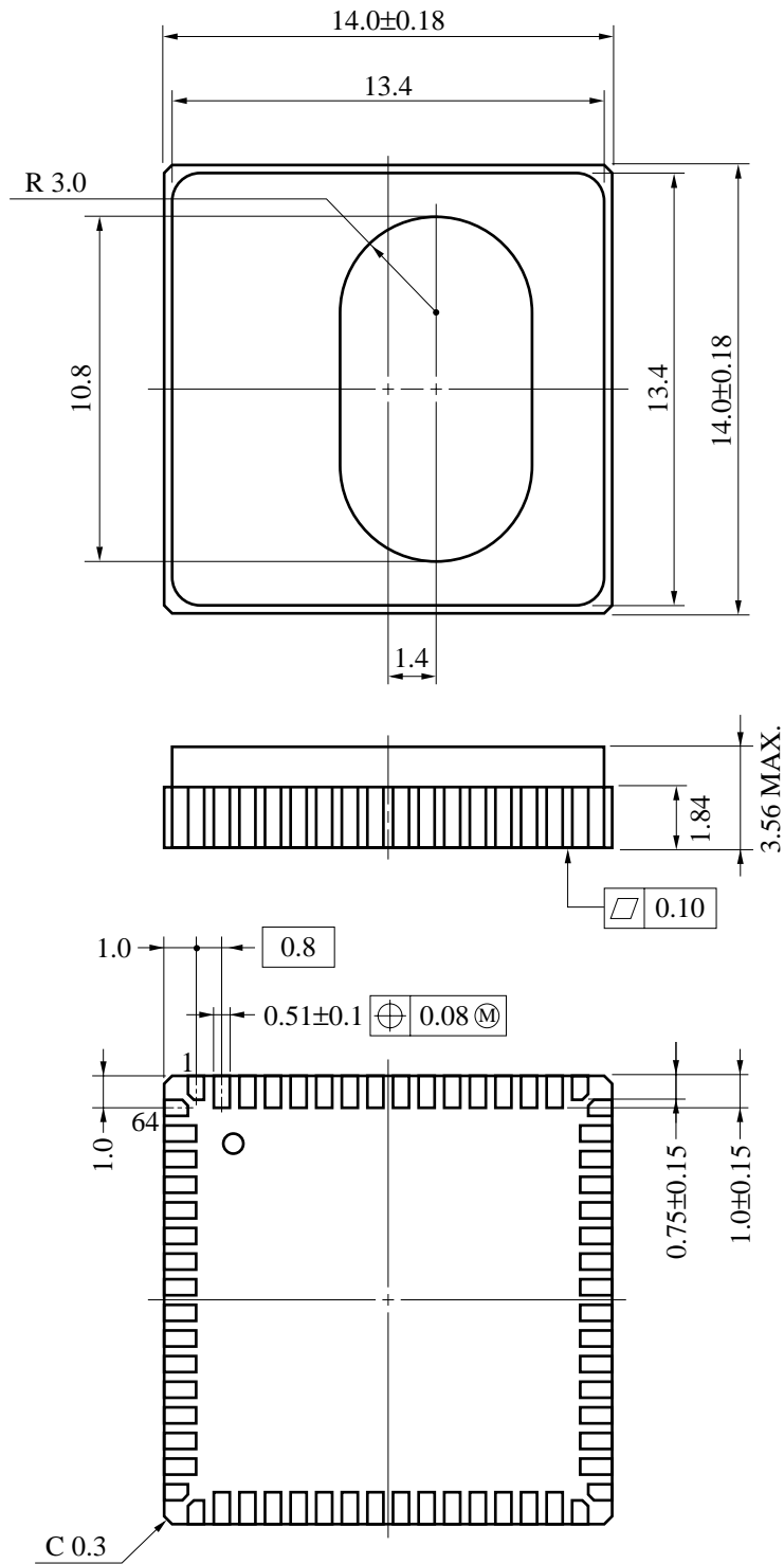
64ピン・セラミック WQFN 外形図 (単位: mm)
