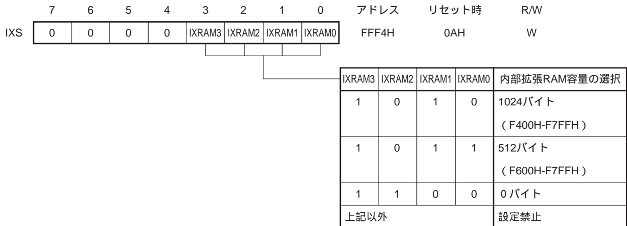
図4 - 1 内部拡張RAMサイズ切り替えレジスタのフォーマット
