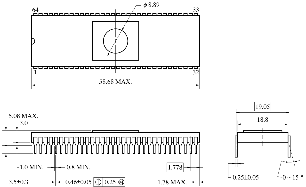
64ピン・セラミック・シュリンク DIP (750 mil) 外形図 (単位: mm)
