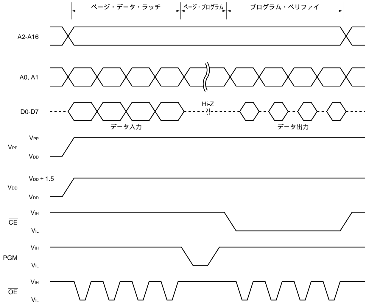
図5-2 ページ・プログラム・モード・タイミング
