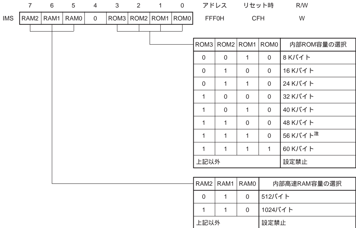
図3 - 1 メモリ・サイズ切り替えレジスタのフォーマット
