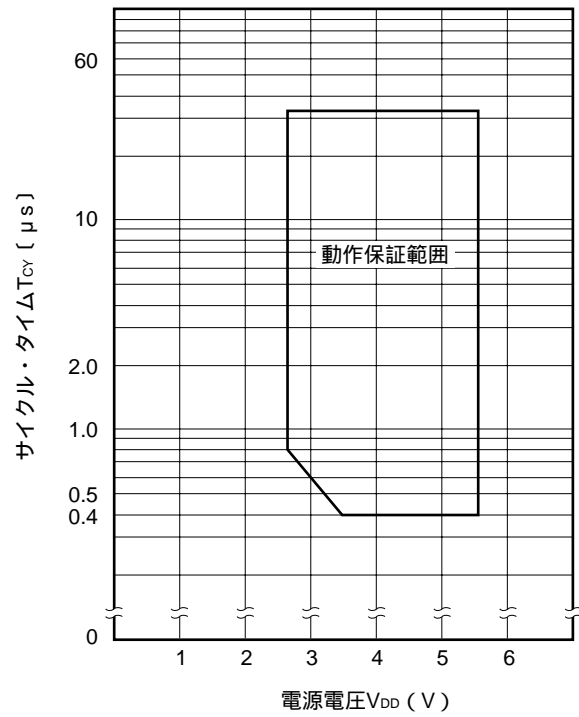
T_{CY} vs V_{DD} (メイン・システム・クロック f_{CX} = f_X 動作時)
