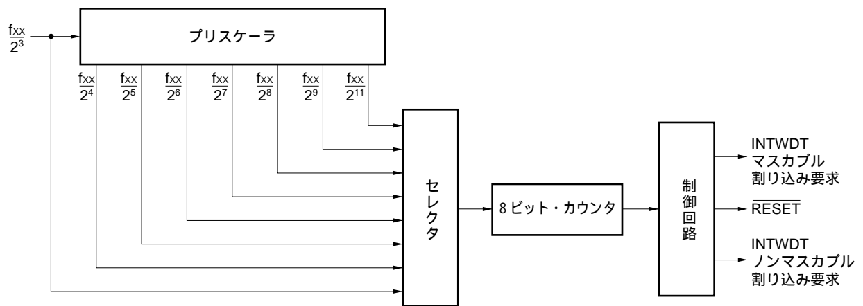
図5 - 6 ウォッチドッグ・タイマのブロック図
