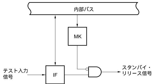
図 6 - 2 テスト機能の基本構成
