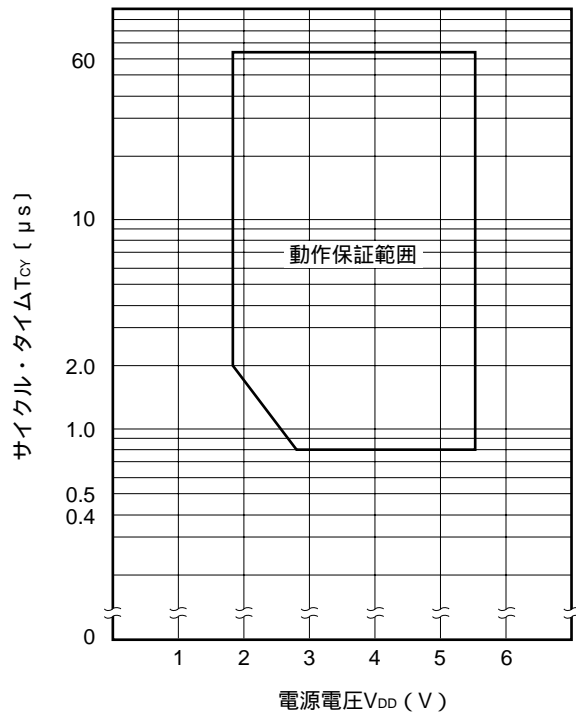
T_{CY} vs V_{DD} (メイン・システム・クロック f_{CX} = f_X/2 動作時)
