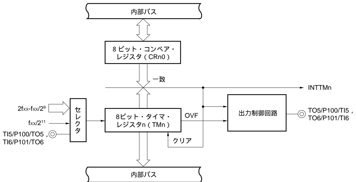
図5 - 4 8ビット・タイマ/イベント・カウンタ5, 6のブロック図
