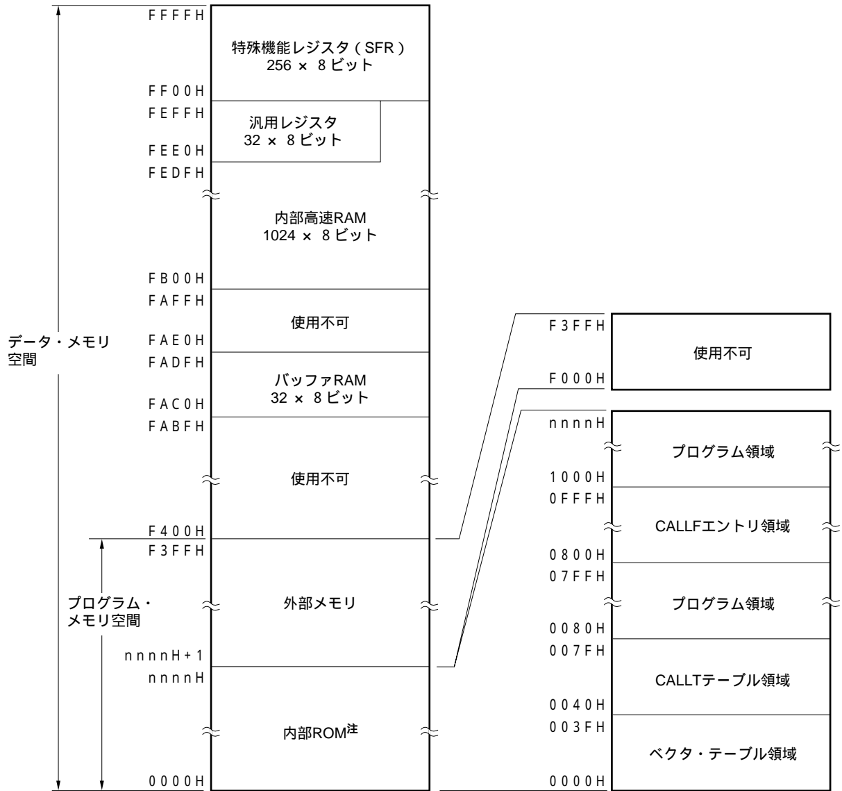
図4 - 1 メモリ・マップ
