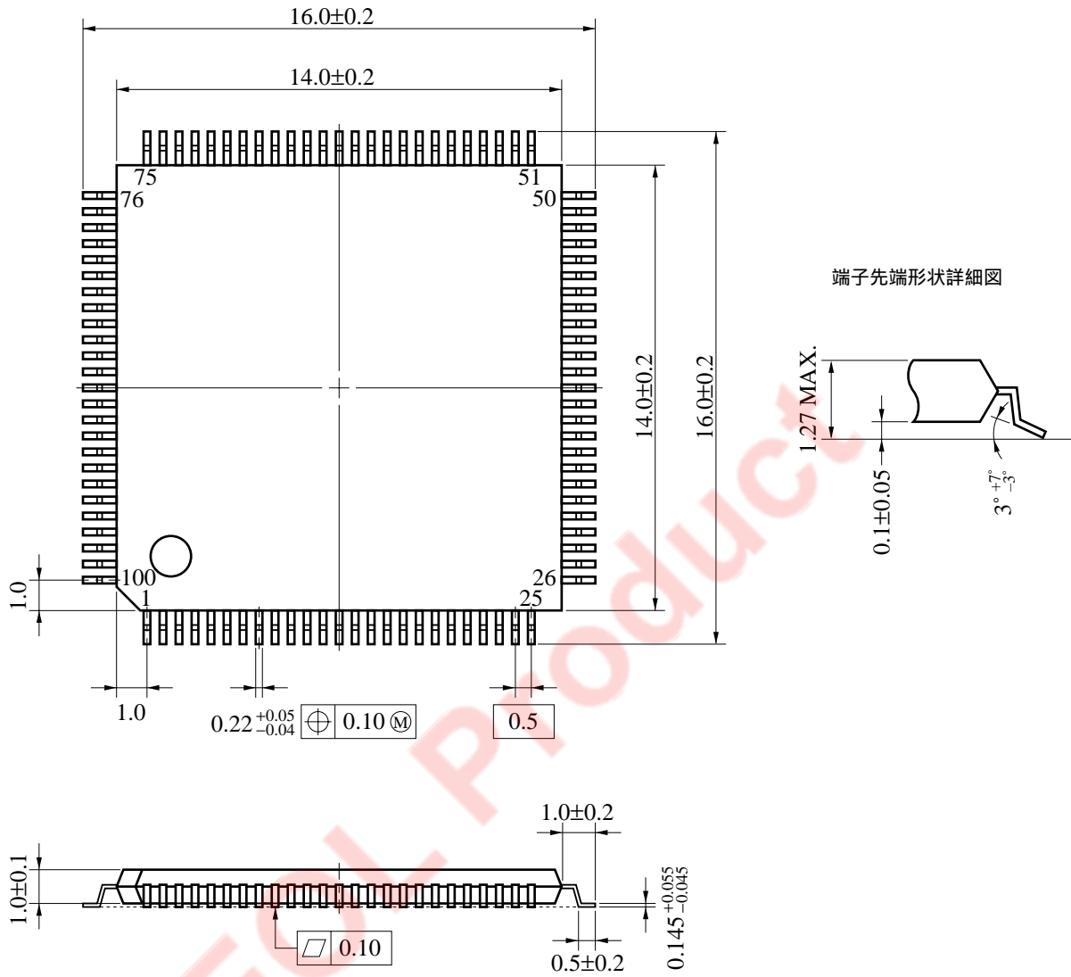
100ピン・プラスチック TQFP (ファインピッチ)( 14)外形図(単位: mm)
