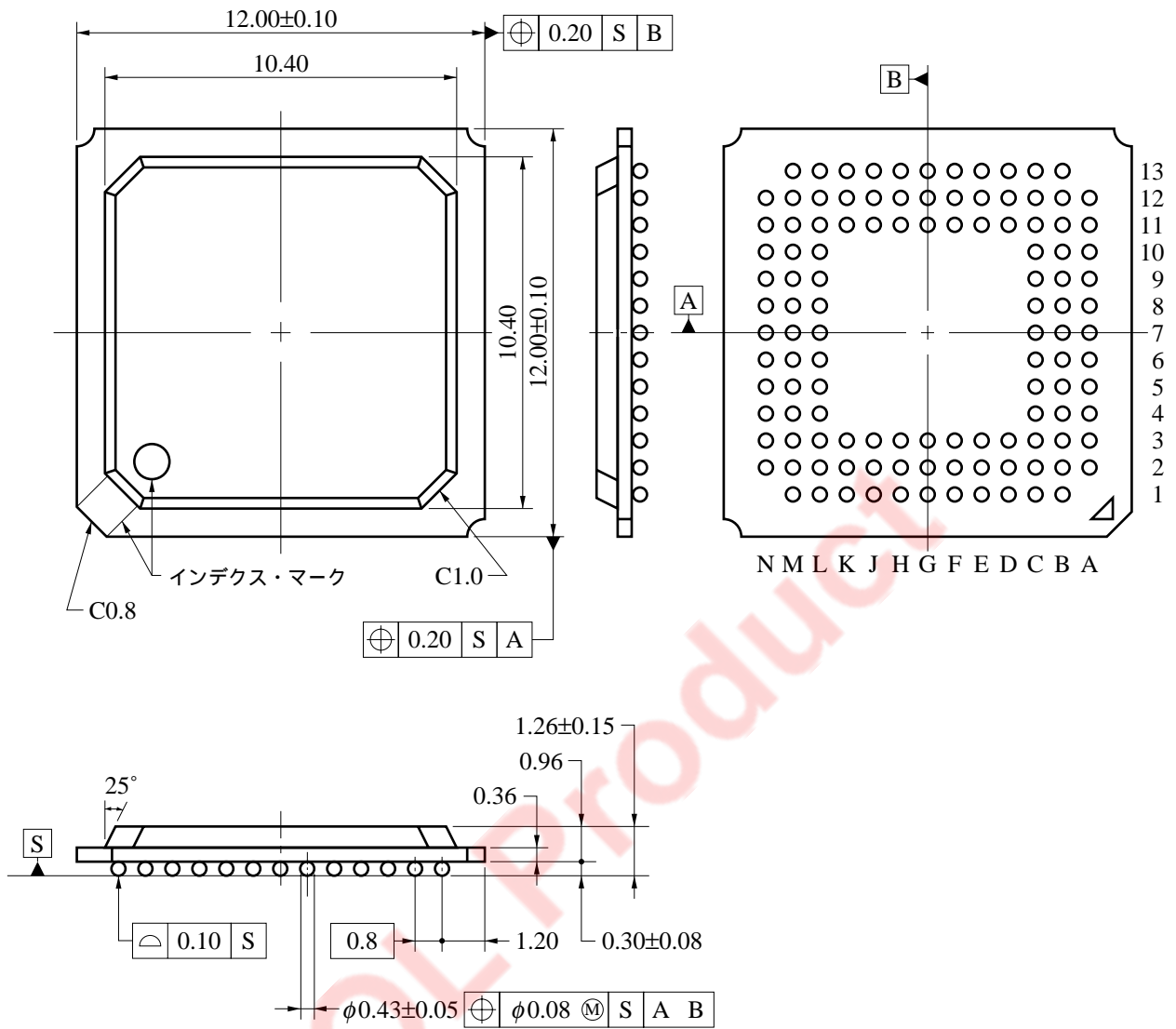
116ピン・ファインピッチ BGA (12x12) 外形図 (単位 : mm)
