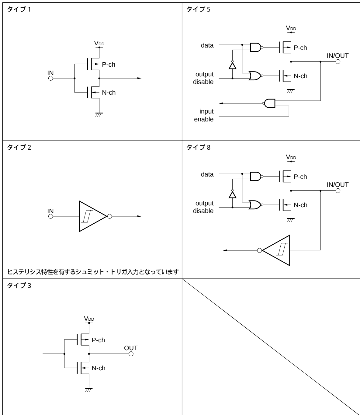
図 2 - 1 端子の入出力回路
