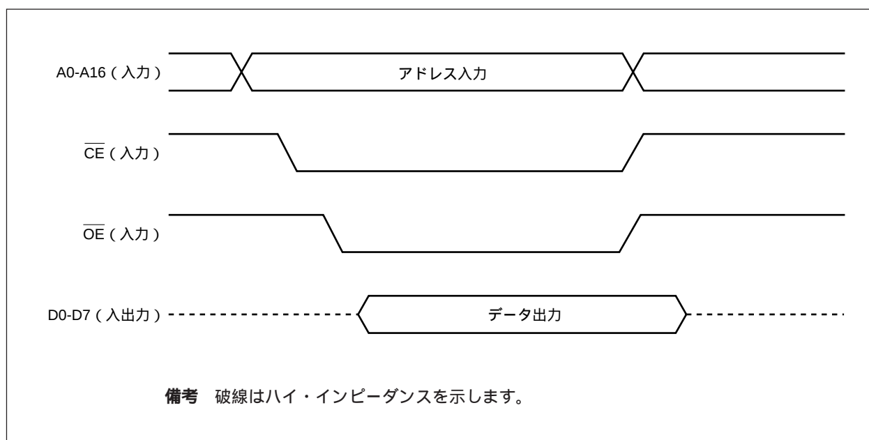
図3 - 5 PROMの読み出しタイミング
