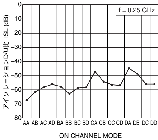
アイソレーションD/U比 vs. ON CHANNEL MODE
