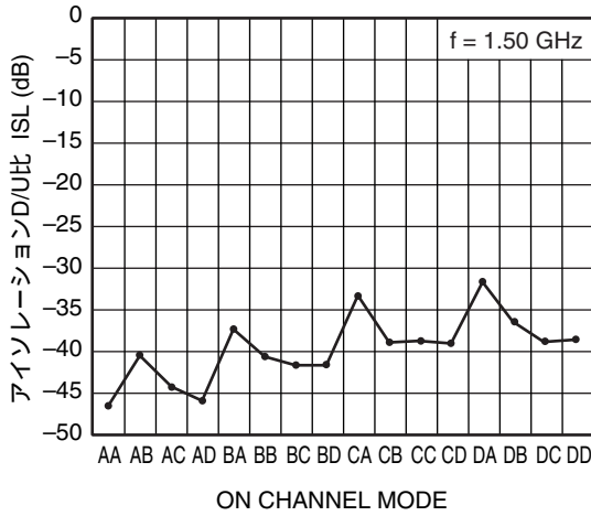
アイソレーションD/U比 vs. ON CHANNEL MODE
