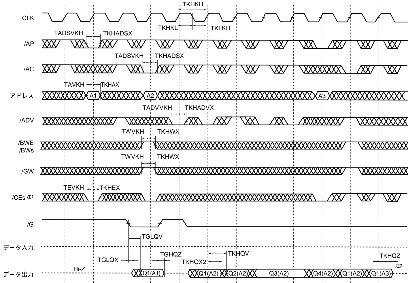
リード・サイクル
