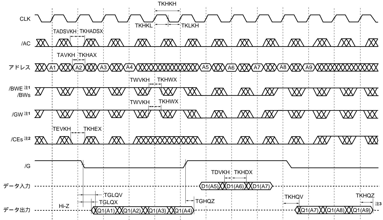
シングル・リード/ライト・サイクル
