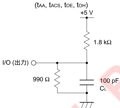
図 1 負荷回路
