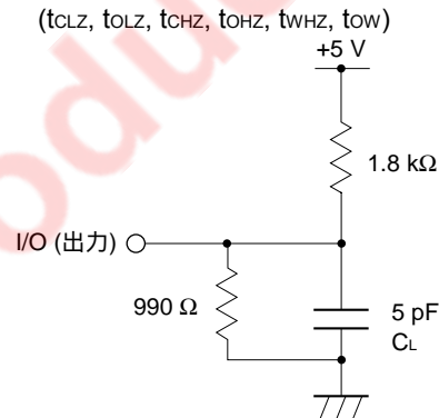
図 2 負荷回路
