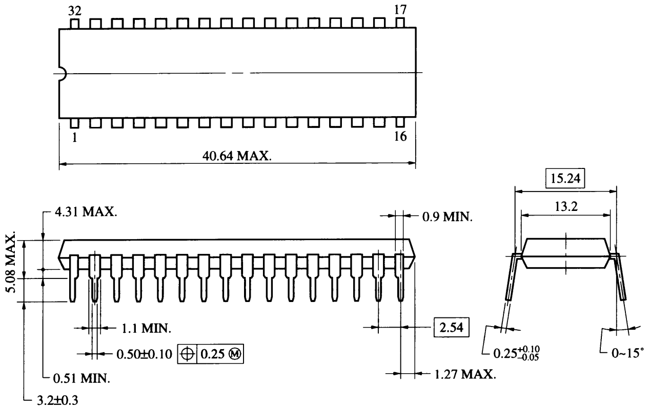
32ピン・プラスチック DIP (600 mil) 外形図 (単位: mm)
