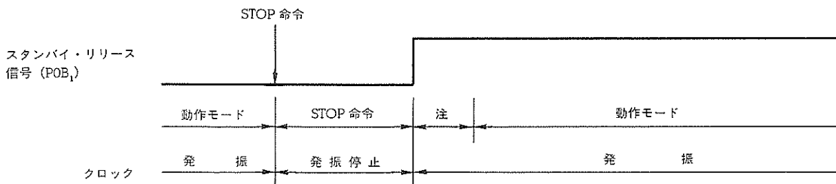
図 7-4 POB 1 端子へのハイ・レベル入力による STOP モードの解除
