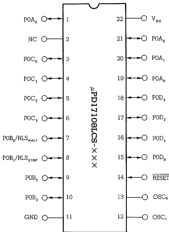
22ピン・プラスチック・シュリンク DIP
