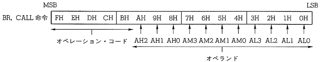
図2-2 16ビット命令の構成
