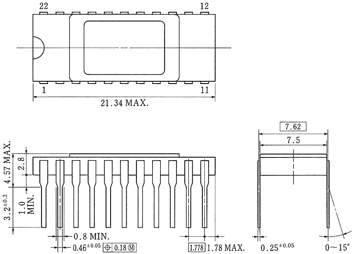
22ピン・セラミック・シュリンク DIP (300 mil) (ES用) 外形図(単位: mm)
