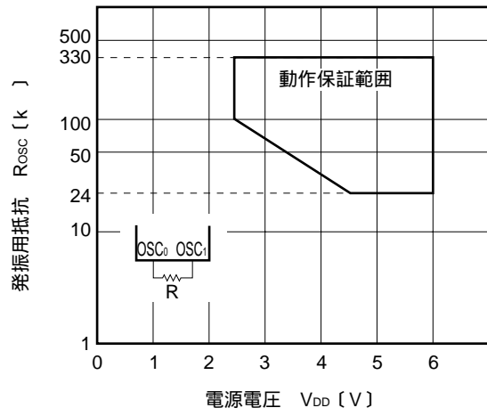
R osc vs V DD 動作保証範囲 (T A = -40 ~ +110 )
