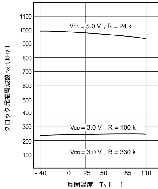
f cc vs T A 特性例
