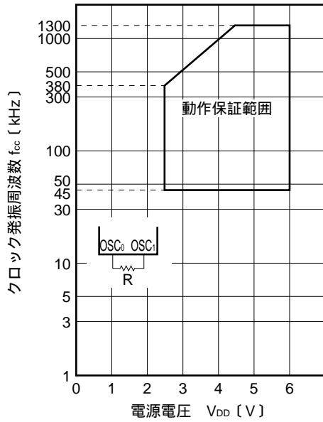
f cc vs V DD 動作保証範囲 (T A = -40 ~ +110 )
