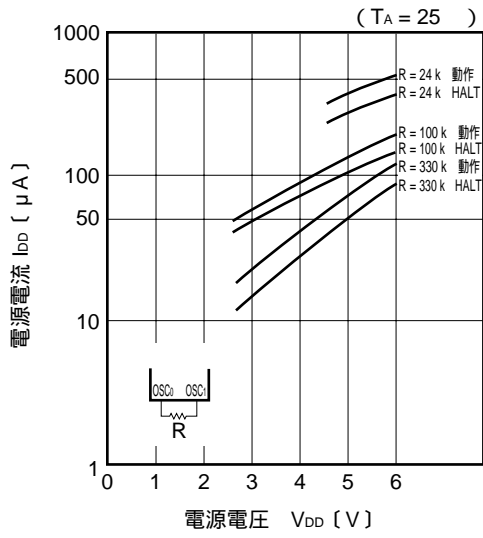
I_{DD} vs V_{DD} 特性例
