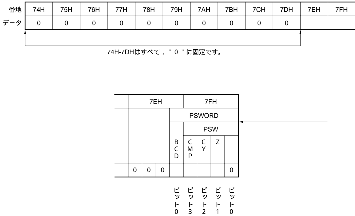
図4 - 2 システム・レジスタ・マップ
