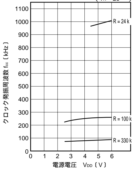
f cc vs V DD 特性例
