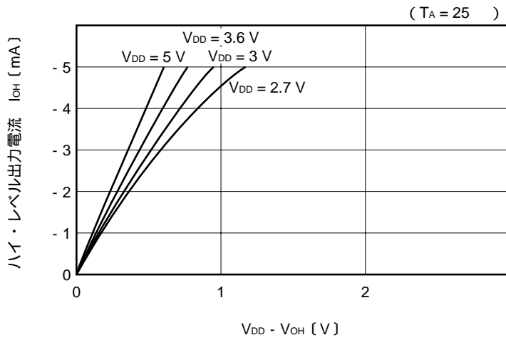
I_{OH} vs ( V_{DD} - V_{OH} ) 特性例
