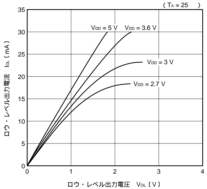
I_{OL} vs V_{OL} 特性例
