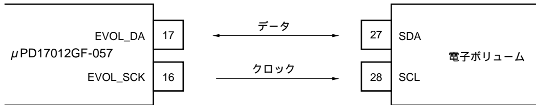
図B - 1 端子接続 (電子ボリューム)
