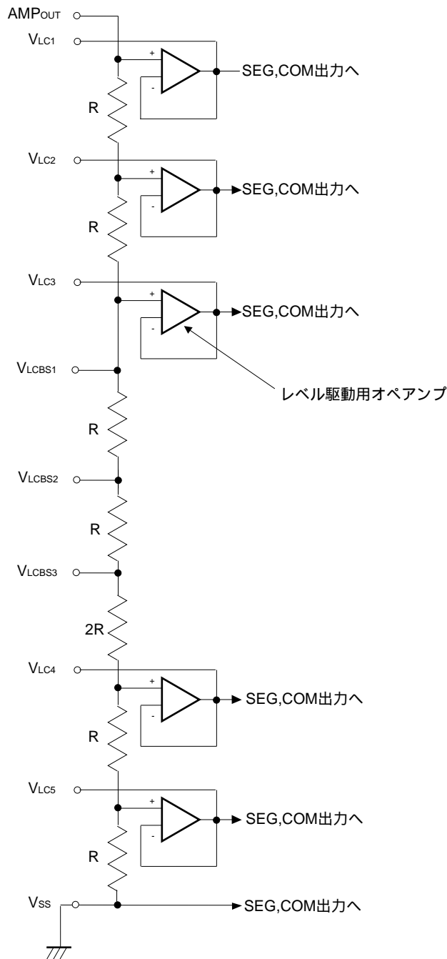
図 4 - 4 基準電圧回路
