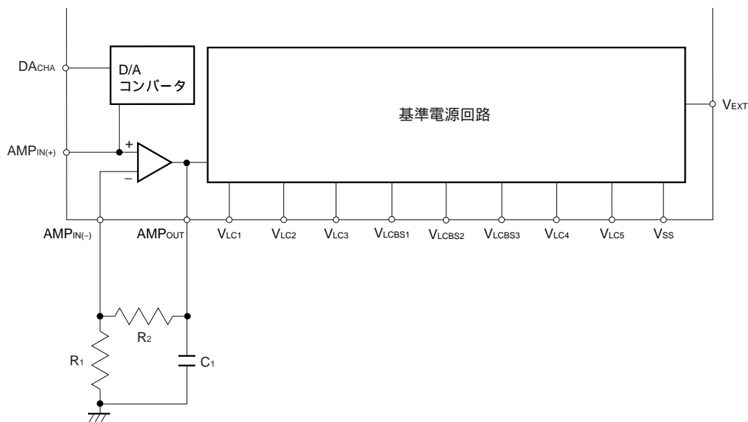
図 3 - 1 電圧制御回路
