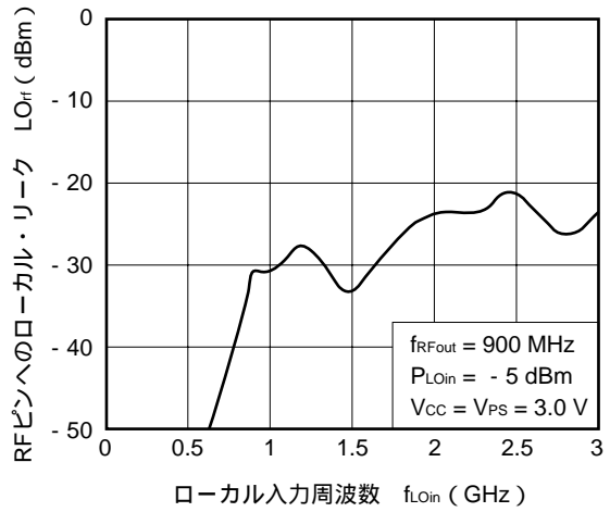
RFピンへのローカル・リーク vs. ローカル入力周波数
