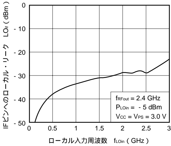
IFピンへのローカル・リーク vs. ローカル入力周波数
