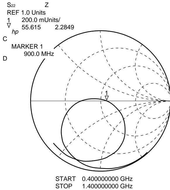
900 MHzマッチング (測定回路図1による)
