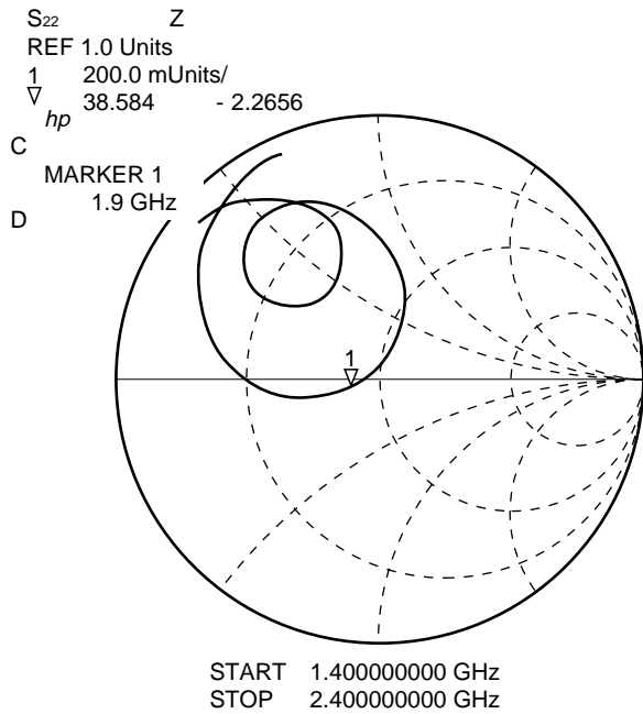
1.9 GHzマッチング (測定回路図2による)
