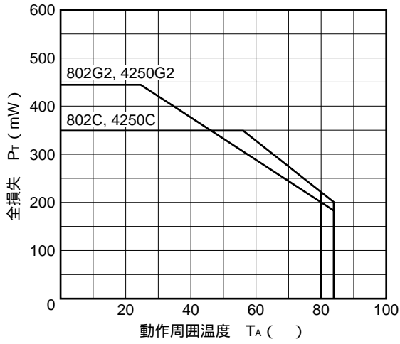
P T - T A 特性 (絶対最大定格)
