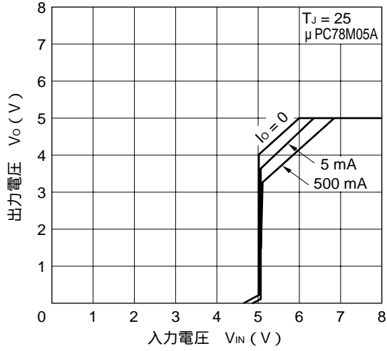
V_o - V_{IN} 特性
