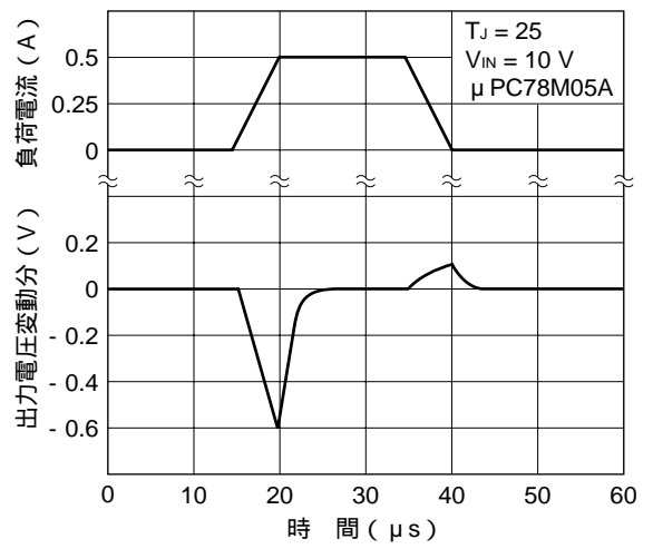
負荷変動応答特性
