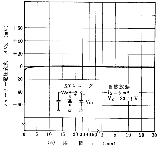
ツェナー電圧経時変化 特性
