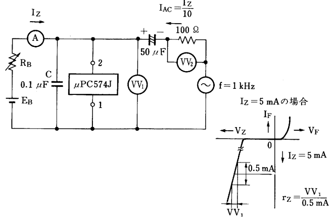
測定回路 2. 動作抵抗 r_z
