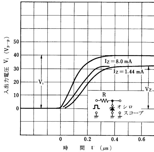
ツェナー電圧過渡 特性
