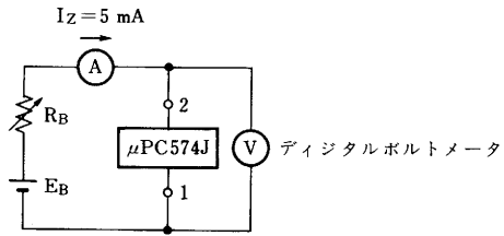
測定回路 1. 安定化電圧 V_Z
