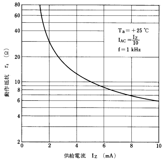
動作抵抗 - 供給電流 特性
