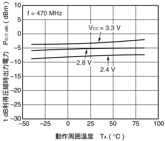
1 dB利得圧縮時出力電力 vs. 動作周囲温度
