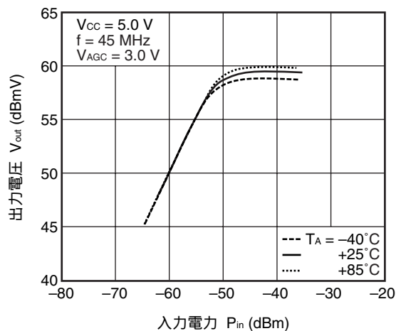
出力電圧 vs. 入力電力
