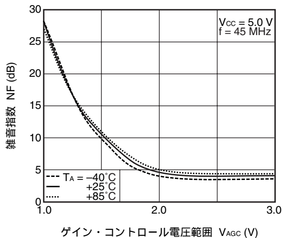
雑音指数 vs. ゲイン・コントロール電圧範囲
