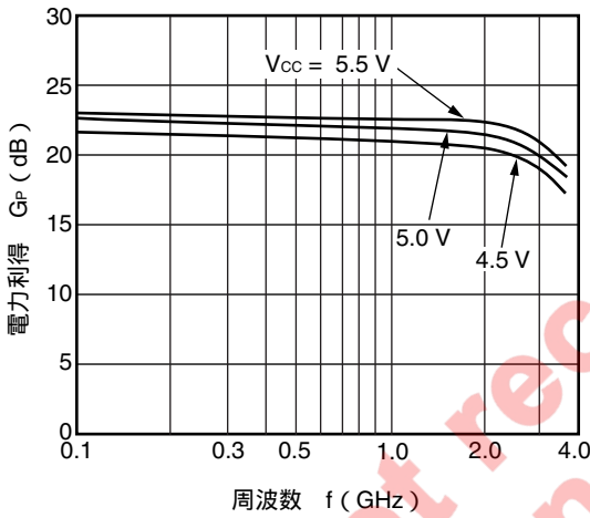
電力利得 vs. 周波数
