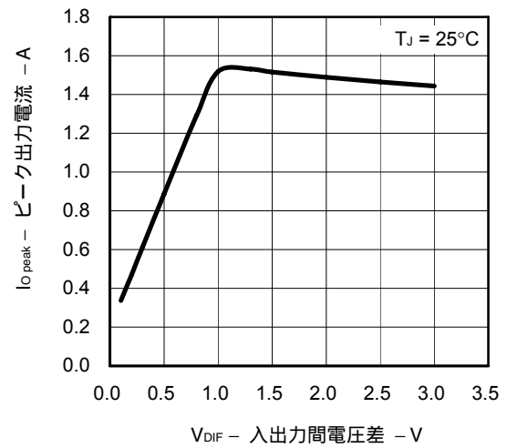
I_{O \text{ peak}} - V_{DIF} 特性 ( \mu PC3005)
