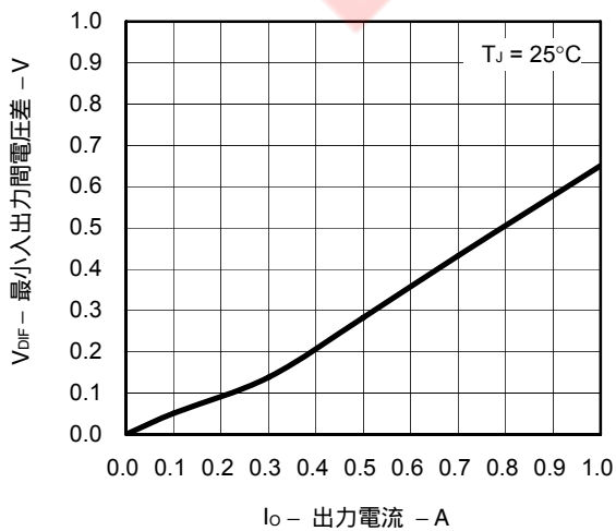
V_{DIF} - I_O 特性 ( \mu PC3005)
