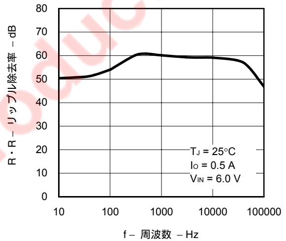
R \cdot R - f 特性 ( \mu PC3005)
