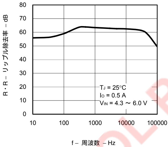
R \cdot R - f 特性 ( \mu PC3033)
