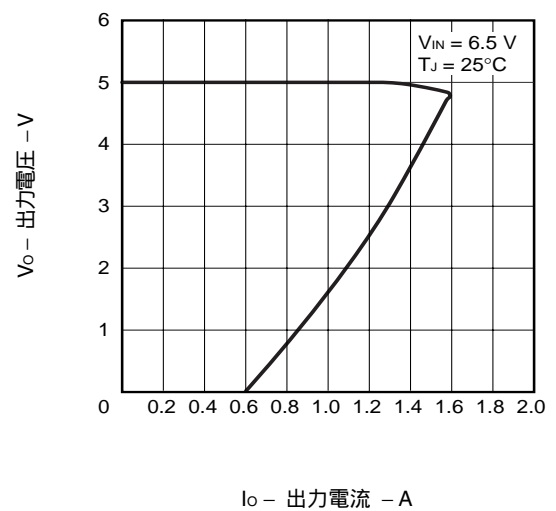
V_O - I_O 特性 ( \mu PC3005)
