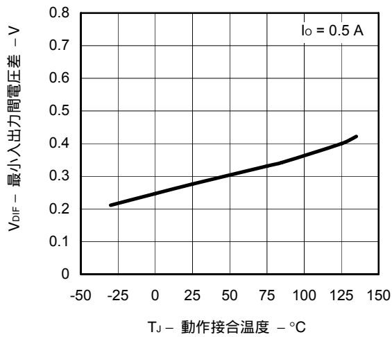
V_{DIF} - T_J 特性 ( \mu PC3005)
