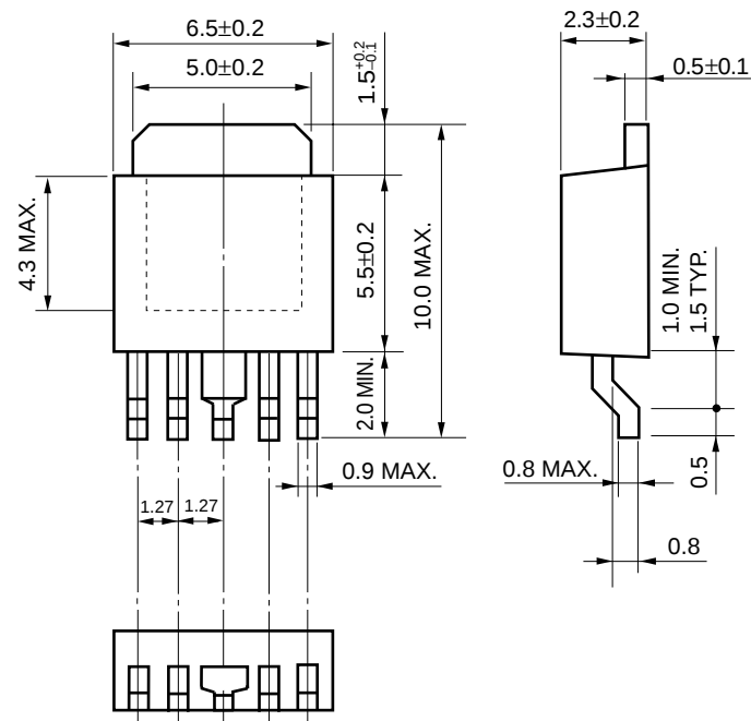
MP-3Z (5ピン) 外形図 (単位: mm)
