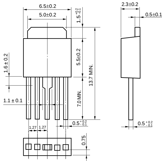
MP-3 (5ピン) 外形図 (単位: mm)
