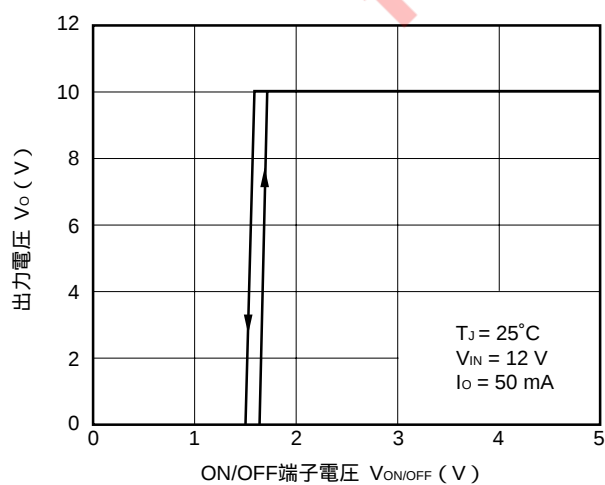
V_O - V_{ON/OFF} 特性
