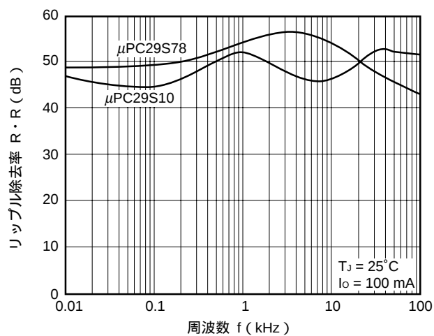
R \cdot R - f 特性
