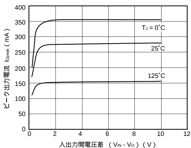
I_{Opeak} - (V_{IN} - V_O) 特性
