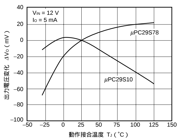
\Delta V_O - T_J 特性
