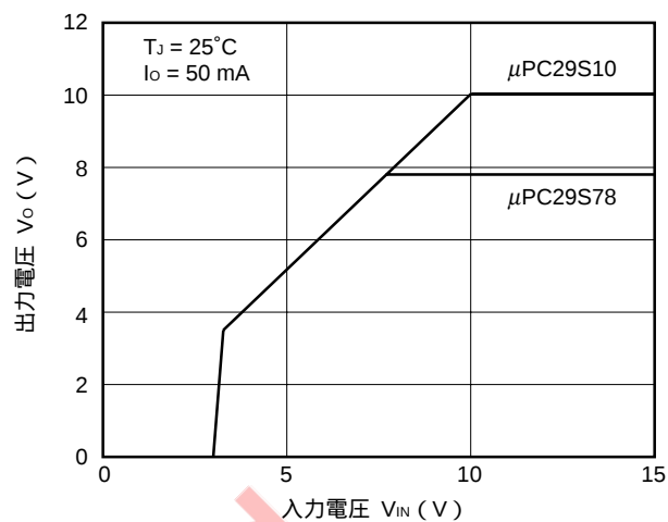
V_O - V_{IN} 特性
