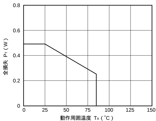
P_T - T_A 特性
