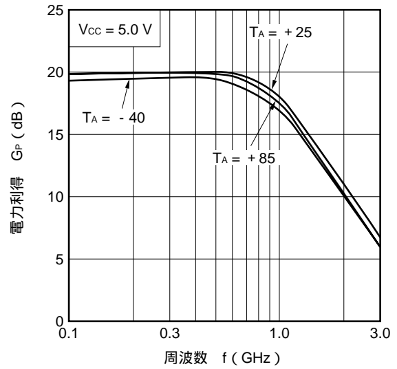
電力利得 vs. 周波数
