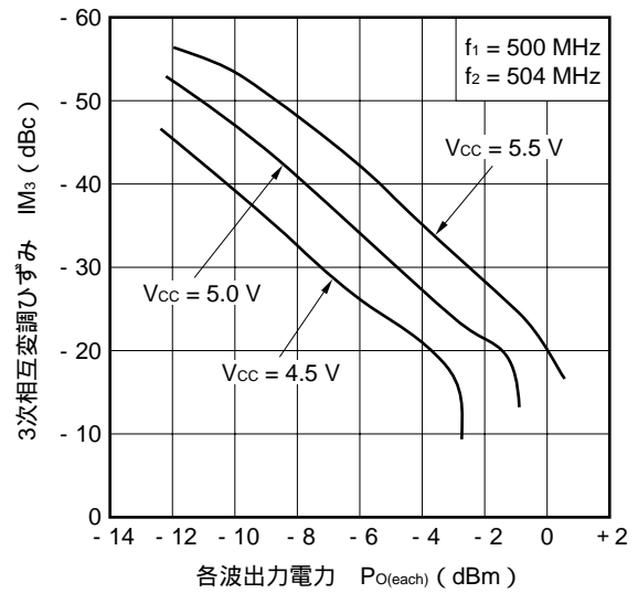
3次相互変調ひずみ vs. 各波出力電力
