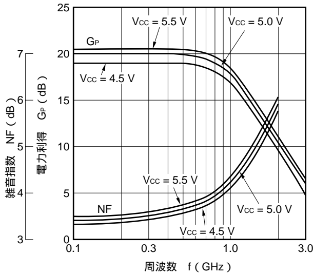
雑音指数, 電力利得 vs. 周波数
