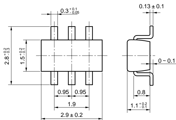
6ピン・ミニモールド外形図(単位: mm)
