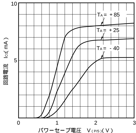
回路電流 vs. パワーセーブ電圧
