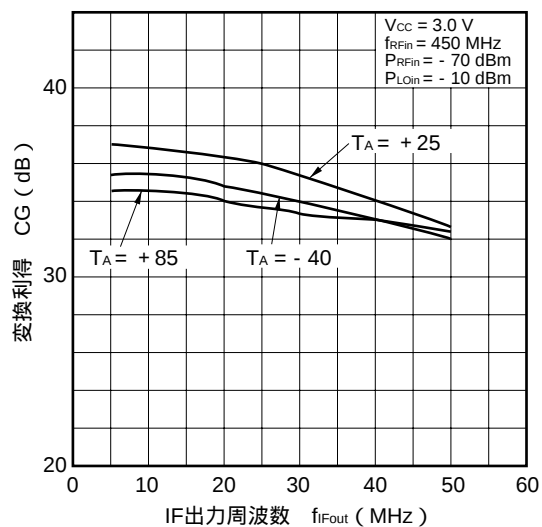
変換利得 vs. IF出力周波数
