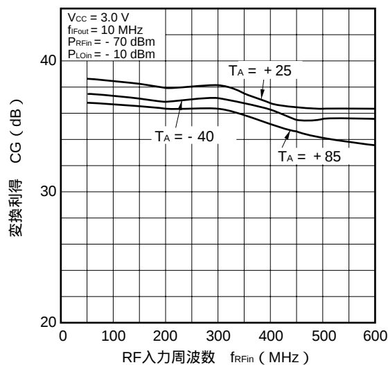
変換利得 vs. RF入力周波数
