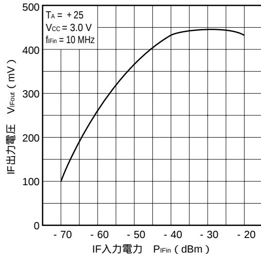
IF出力電圧 vs. IF入力電力
