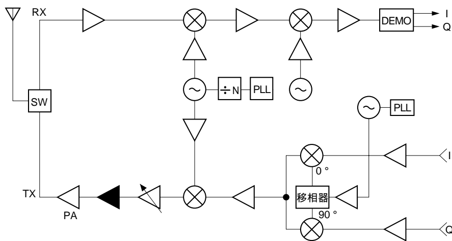
◀ : \mu PC2762T, 2763T 推奨部分
