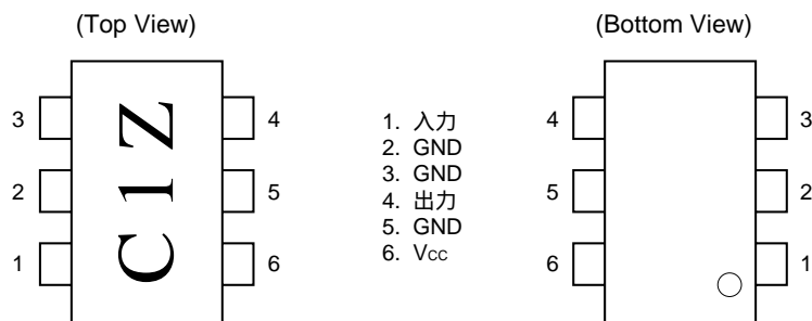
捺印は μPC2762Tの例
