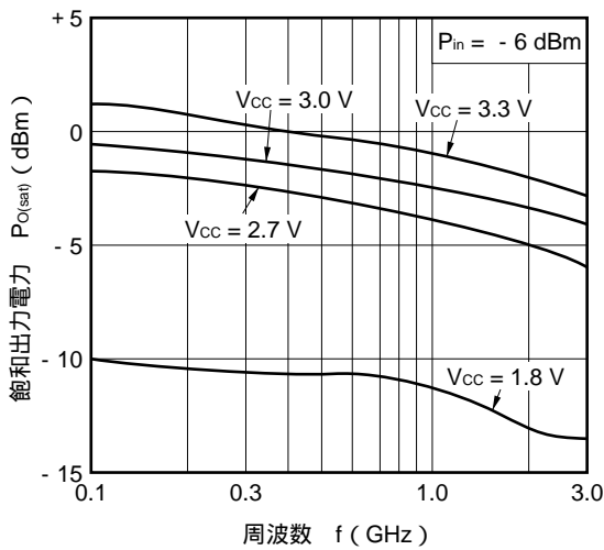
飽和出力電力 vs. 周波数
