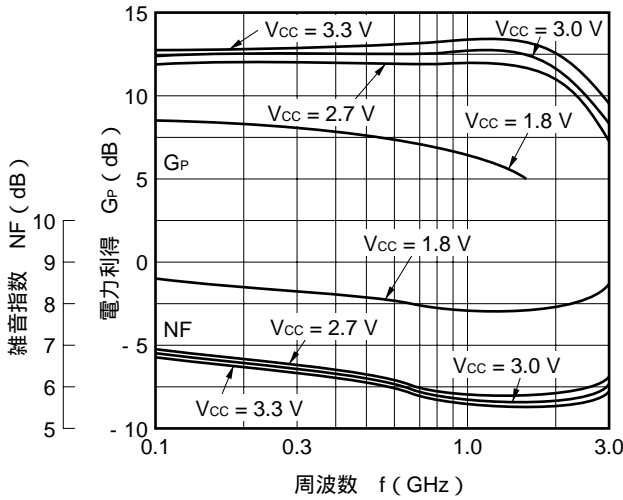
雑音指数, 電力利得 vs. 周波数
