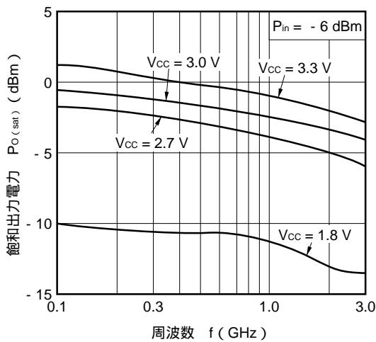
P o(sat) - f 特性
