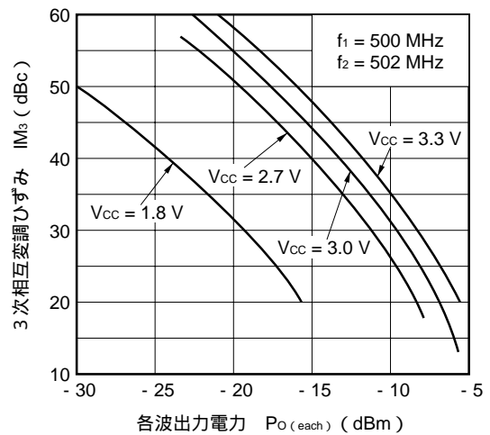
IM 3 - P o(sat) 特性
