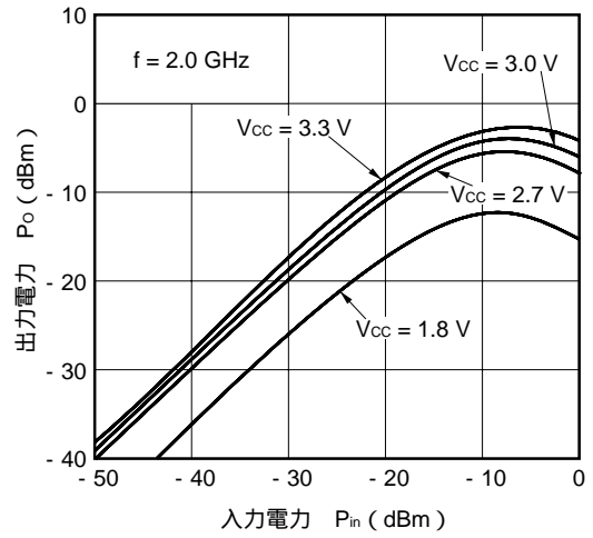
P o - P in 特性
