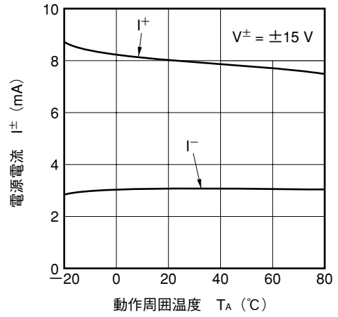
I^\pm - T_A 特性
