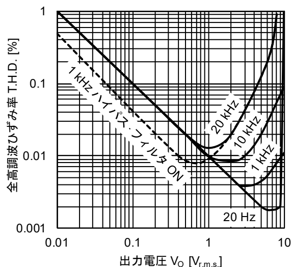
ひずみ率特性
