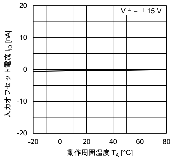
I_{IO} - T_A 特性
