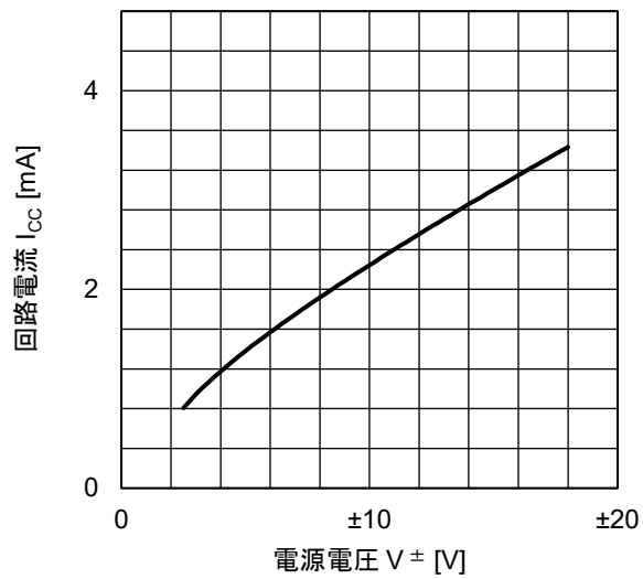
I_{CC} - V^{\pm} 特性
