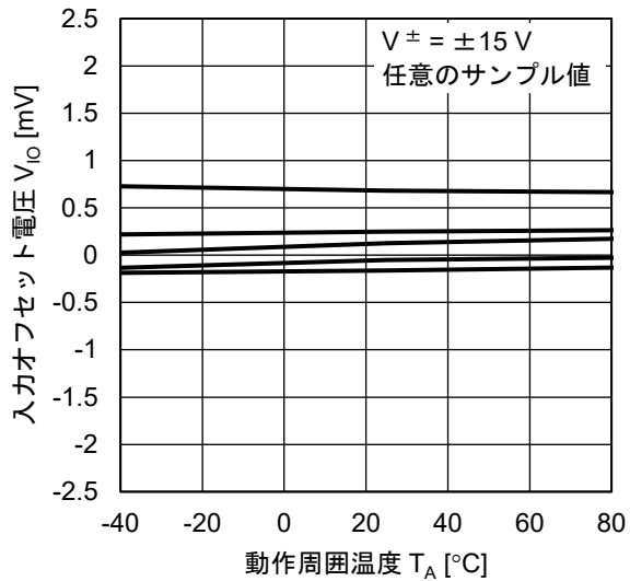
V_{IO} - T_A 特性
