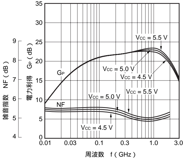
電力利得, 雑音指数 vs. 周波数
