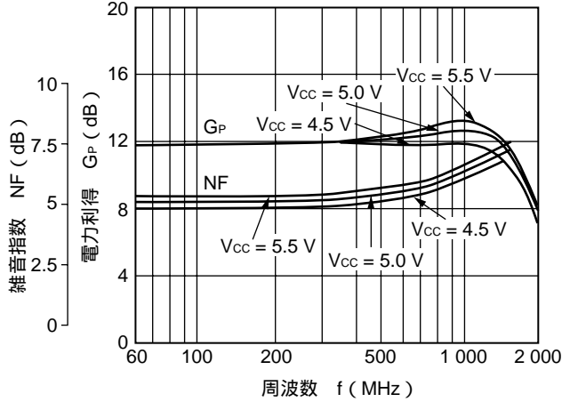
雑音指数, 電力利得 vs. 周波数
