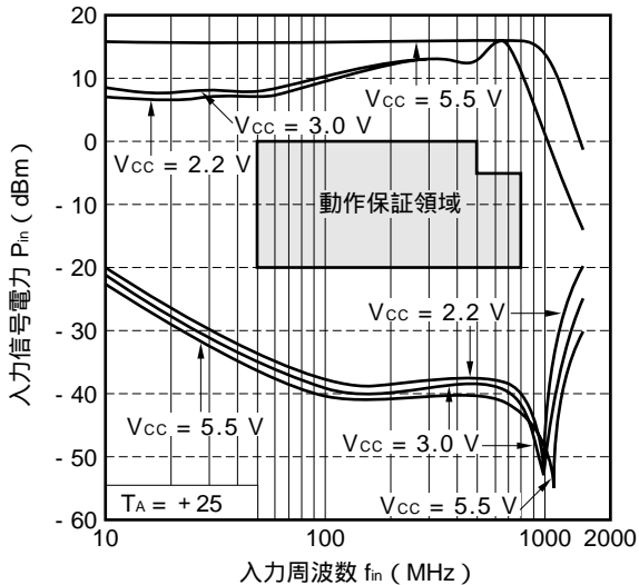
入力信号電力 vs. 入力周波数
