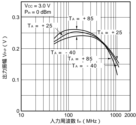
出力振幅 vs. 入力周波数
