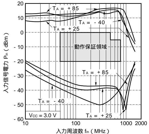
入力信号電力 vs. 入力周波数
