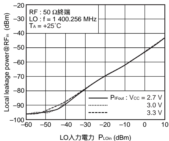
Local leakage power@RF<sub>in</sub> vs. LO入力電力
