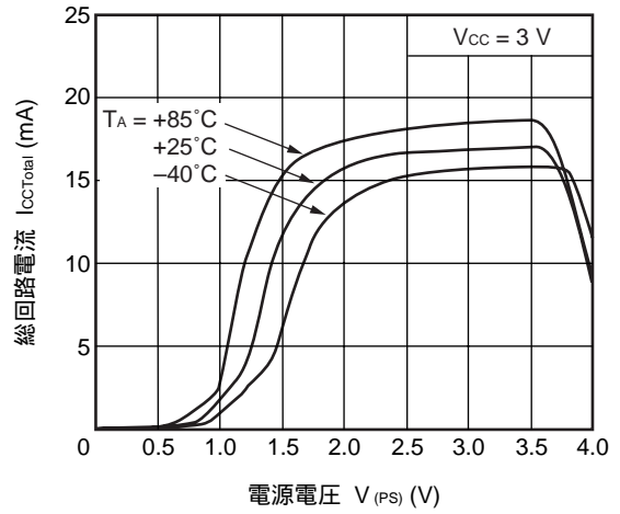
総回路電流 vs. 電源電圧 V_{(PS)}
