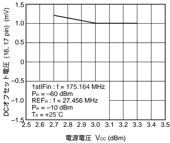
DCオフセット電圧 (16, 17 pin) vs. 電源電圧
