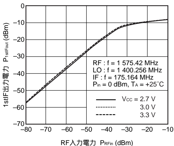
1stIF出力電力 vs. RF入力電力
