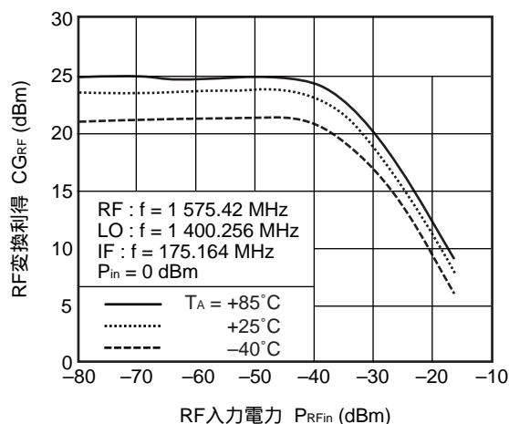
RF変換利得 vs. RF入力電力
