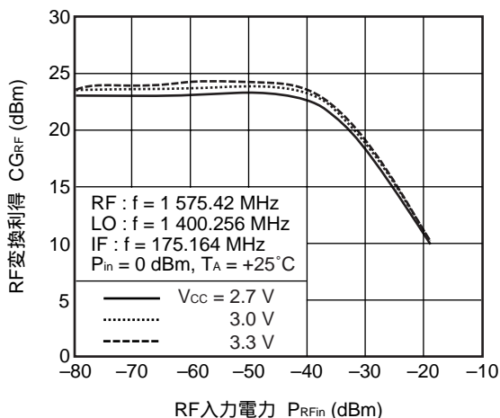
RF変換利得 vs. RF入力電力
