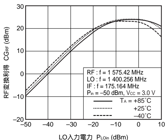
RF変換利得 vs. LO入力電力
