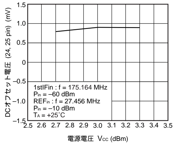
DCオフセット電圧 (24, 25 pin) vs. 電源電圧
