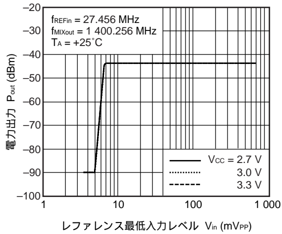
Pout@RF MIXout vs. レファレンス最低入力レベル
