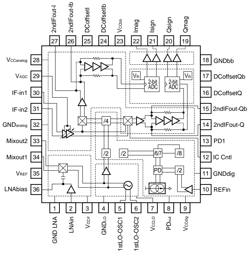
端子接続および内部ブロック図
