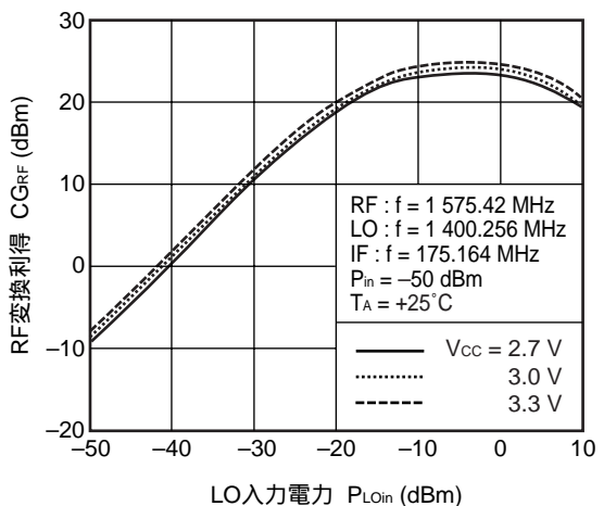
RF変換利得 vs. LO入力電力
