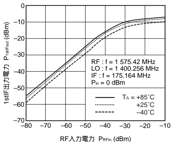
1stIF出力電力 vs. RF入力電力
