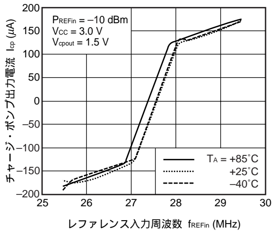
チャージ・ポンプ出力電流 vs. レファレンス入力周波数
