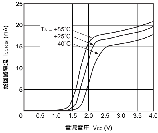
総回路電流 vs. 電源電圧
