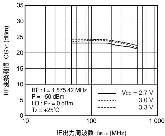
RF変換利得 vs. IF出力周波数
