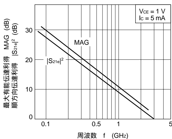
最大有能伝達利得 順方向伝達利得 vs. 周波数
