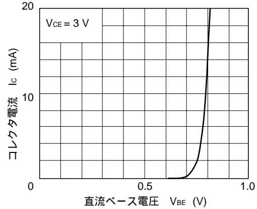
コレクタ電流 vs. 直流ベース電圧
