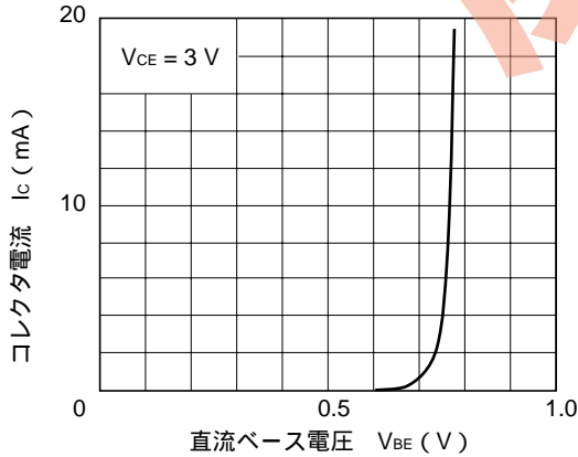
コレクタ電流 vs. 直流ベース電圧
