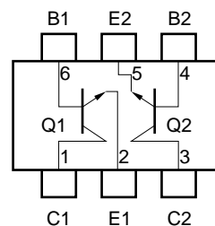
端子接続（Top View）
