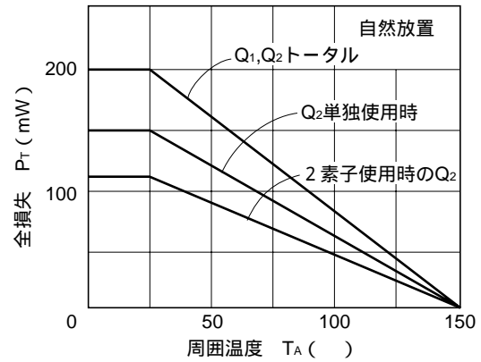
全損失 vs. 周囲温度
