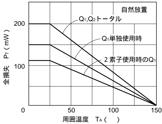
全損失 vs. 周囲温度
