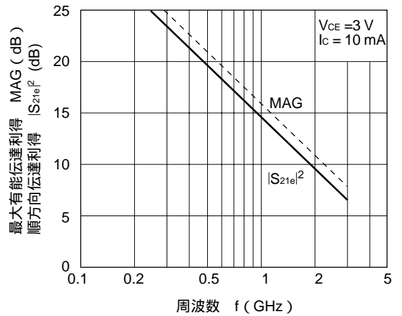
最大有能伝達利得 順方向伝達利得 vs. 周波数
