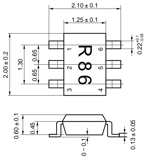
端子接続（Top View）
