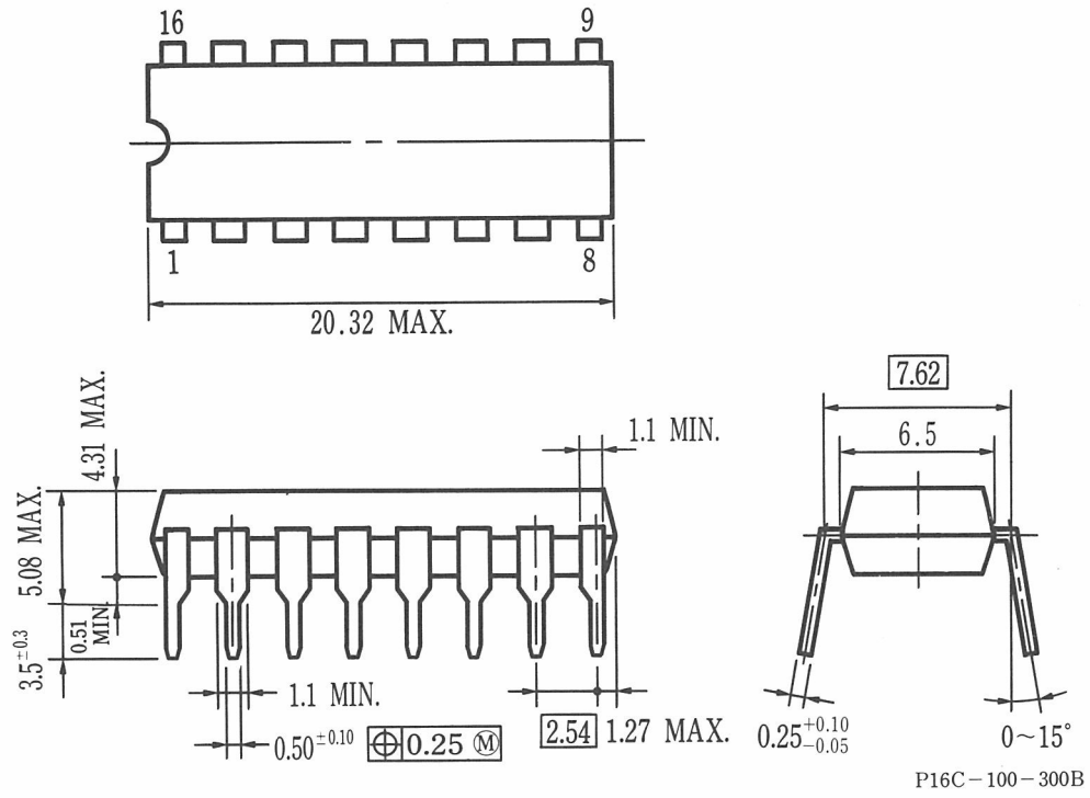
16ピン・プラスチック・シュリンク DIP (300 mil) 外形図(単位: mm)
