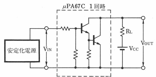
V_o - V_i 特性測定回路
