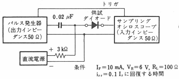
t_{rr} 測定回路
