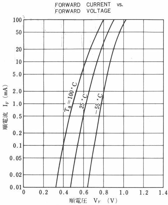
特性曲線 ( T_a = 25^\circ\text{C} )
