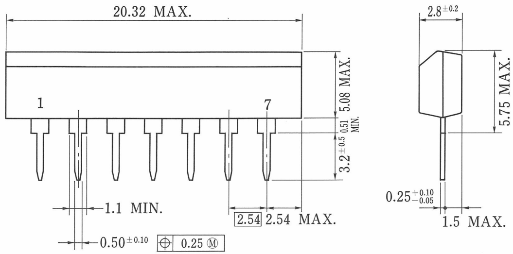
7ピン・プラスチック・スリム SIP 外形図 (単位: mm)
