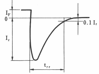
ダイオードに流れる電流波形
